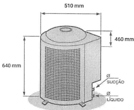
UNIDADE EXTERNA (CONDENSADORA)
