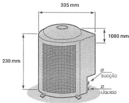
UNIDADE EXTERNA (CONDENSADORA)
