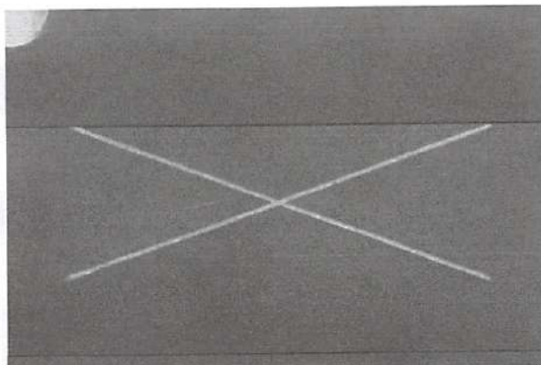
Terceiro teste de aderência do CPS 1. Classificação Y_0/X_0 (isento de destacamento).
