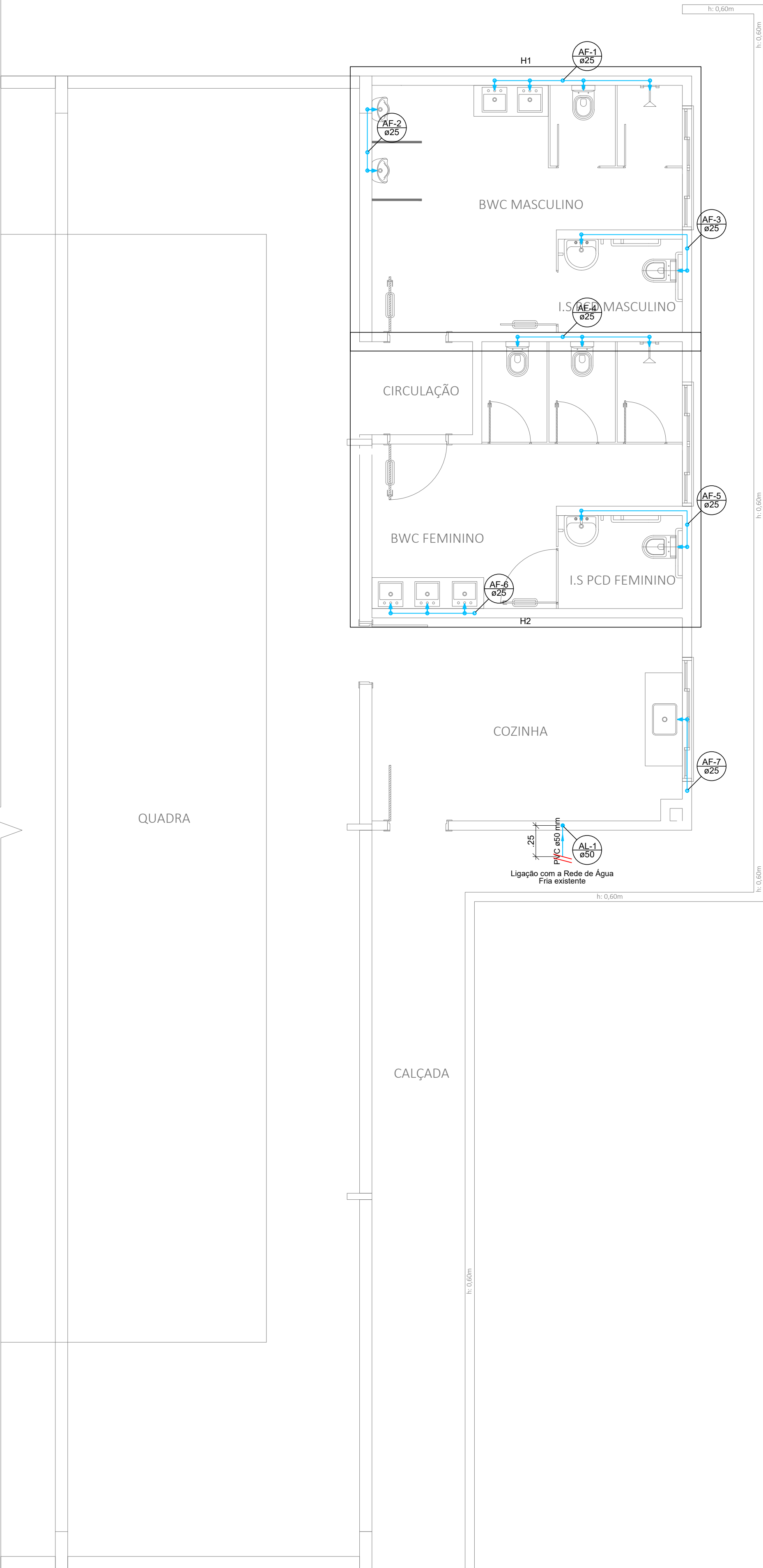
PLANTA BAIXA - HIDRÁULICA ESCALA: 1:50
