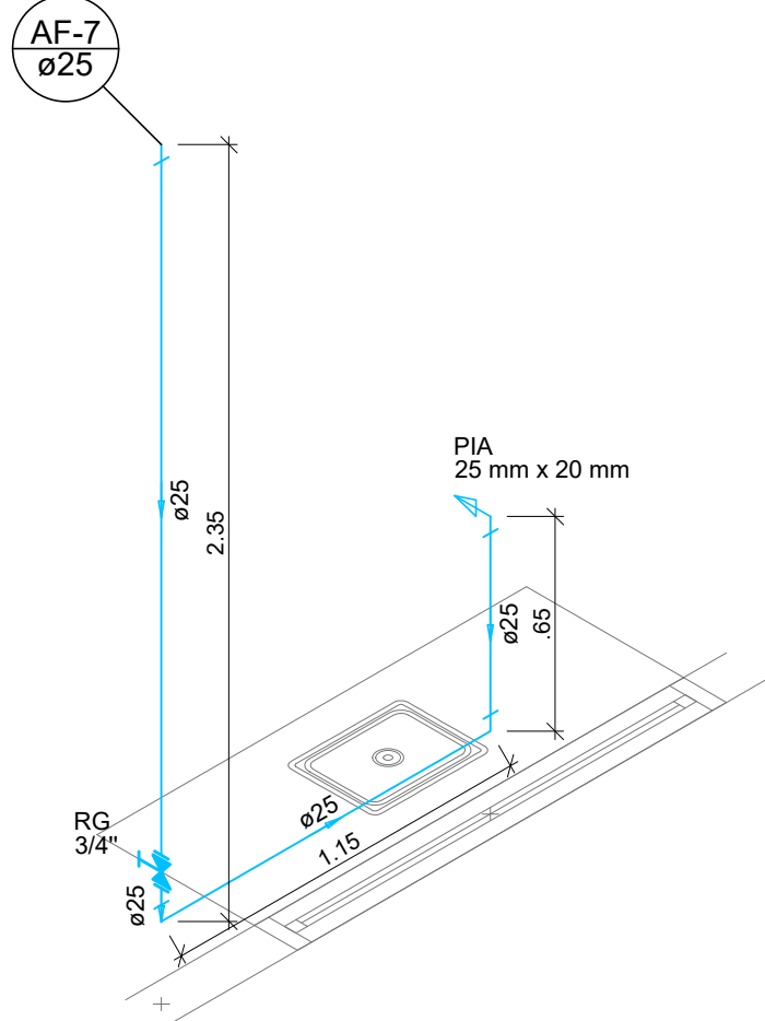
Detalhe H03 Escala 1:25
