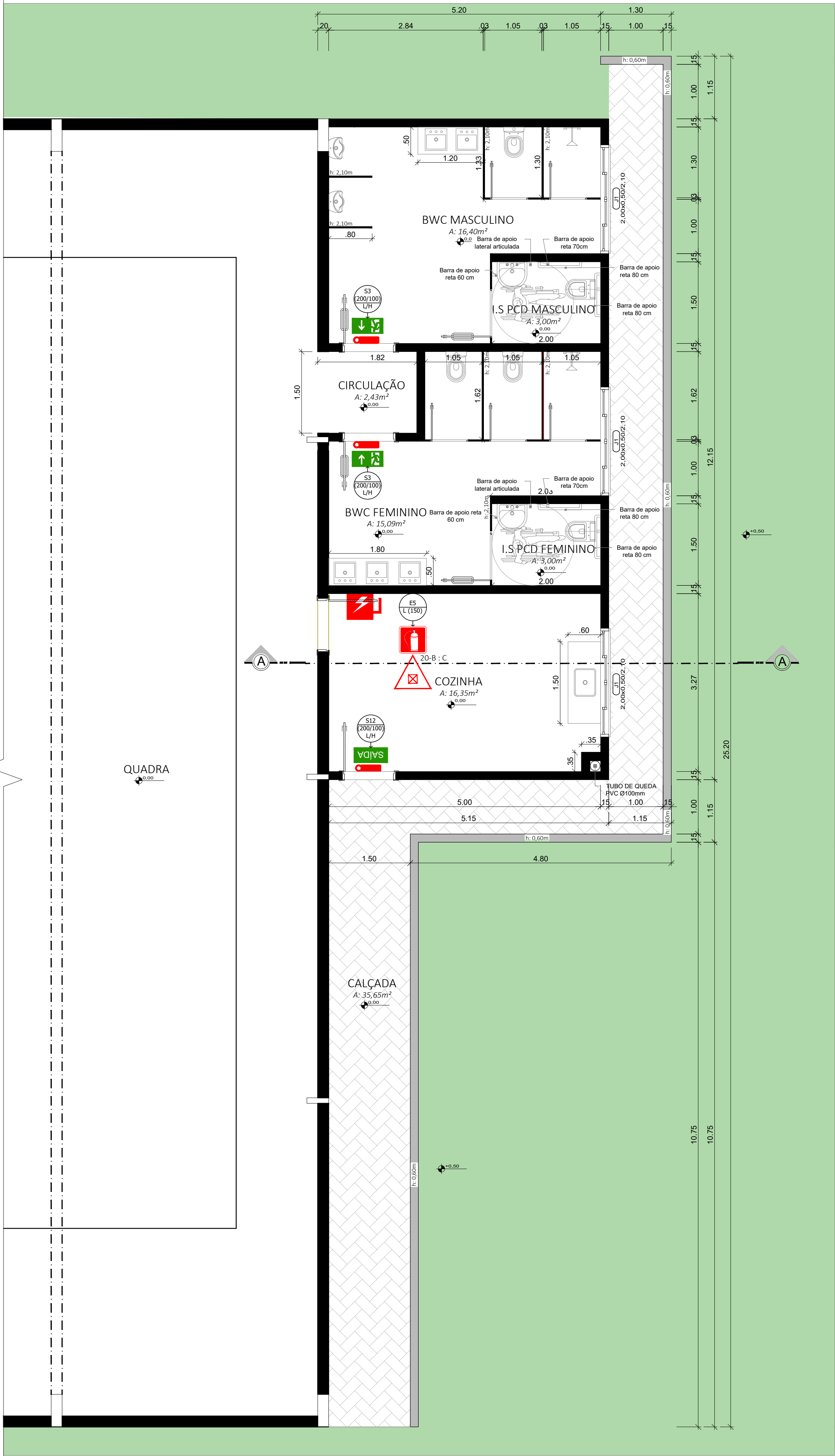
PLANTA BAIXA ÁREA A SER AMPLIADA: 62,57m² ESCALA: 1:50
