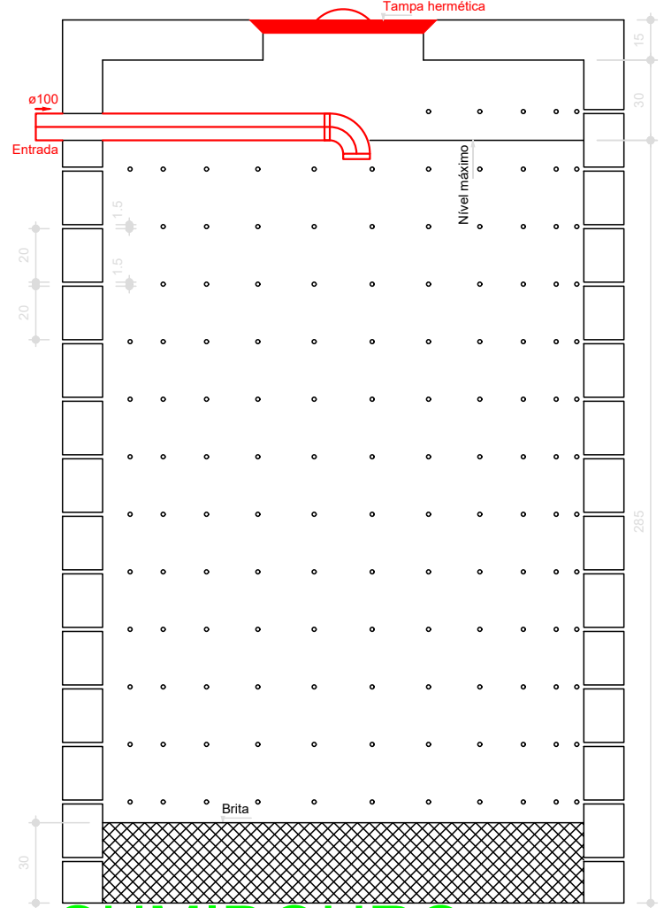
SUMIDOURO CORTE - ESC. 1:25
