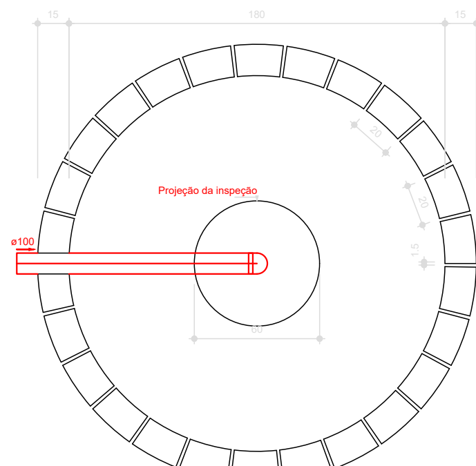
SUMIDOURO PLANTA BAIXA - ESC. 1:25
