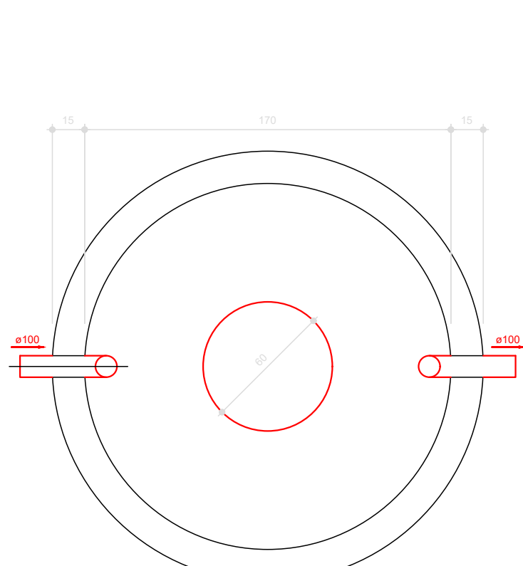
TANQUE SÉPTICO PLANTA BAIXA - ESC. 1:25
