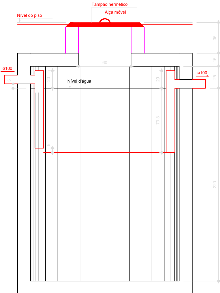
TANQUE SÉPTICO CORTE - ESC. 1:25
