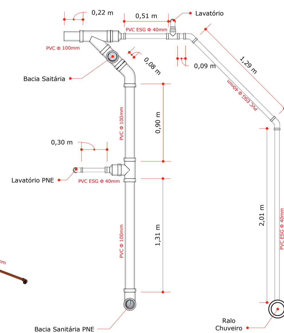
13 PLANTA BAIXA SANITÁRIA BWC MASC. S/ ESCALA
