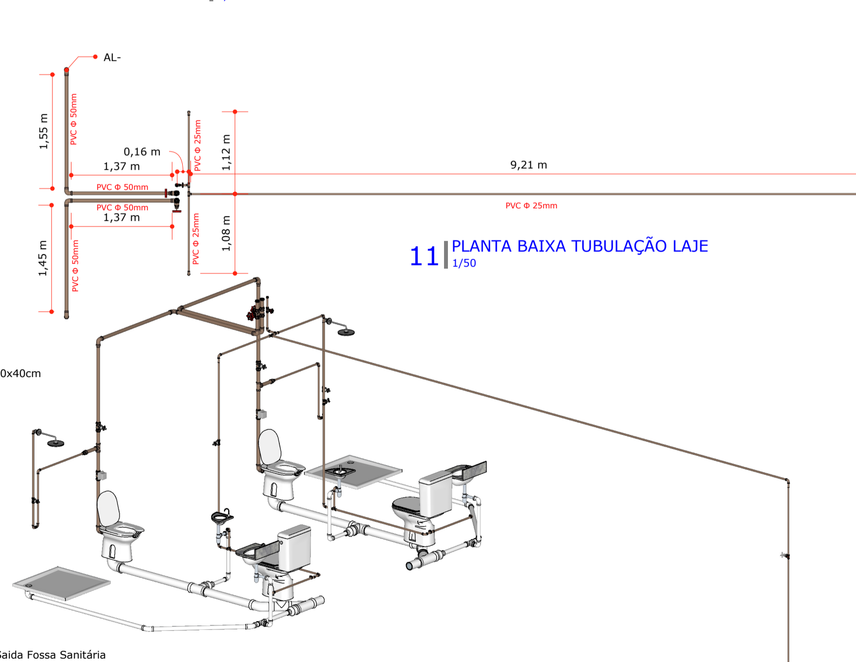
12 DETALHE ISOMETRICO AL-4 - ÁGUA FRIA S/ ESCALA
