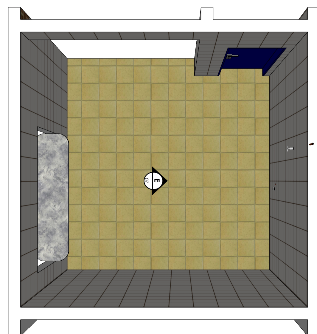
15 PLANTA BAIXA COZINHA ESCALA 1/50
