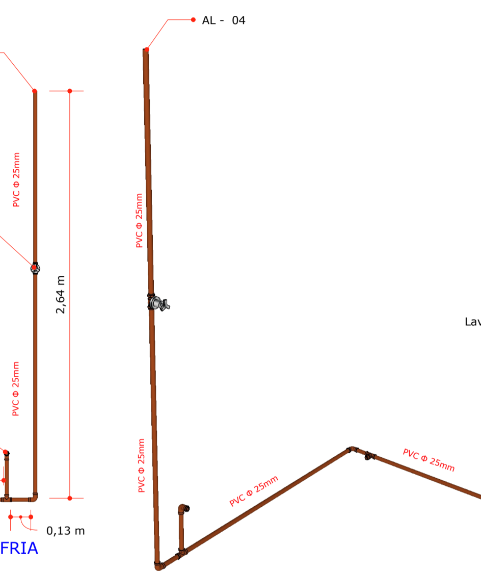
12 DETALHE ISOMETRICO AL-4 - ÁGUA FRIA S/ ESCALA
