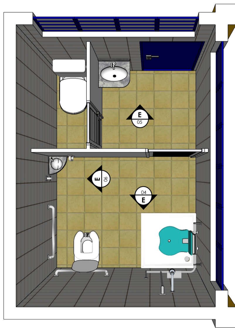
08 PLANTA BAIXA BANHEIRO MASCULINO ESCALA 1/50
