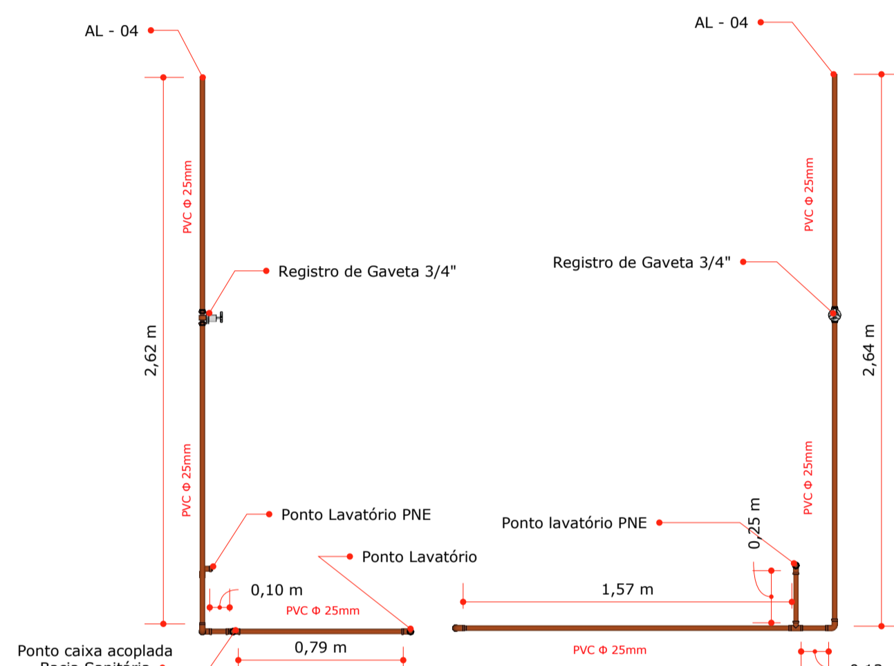
11 ELEVAÇÃO 06 - ÁGUA FRIA ESCALA 1/50
