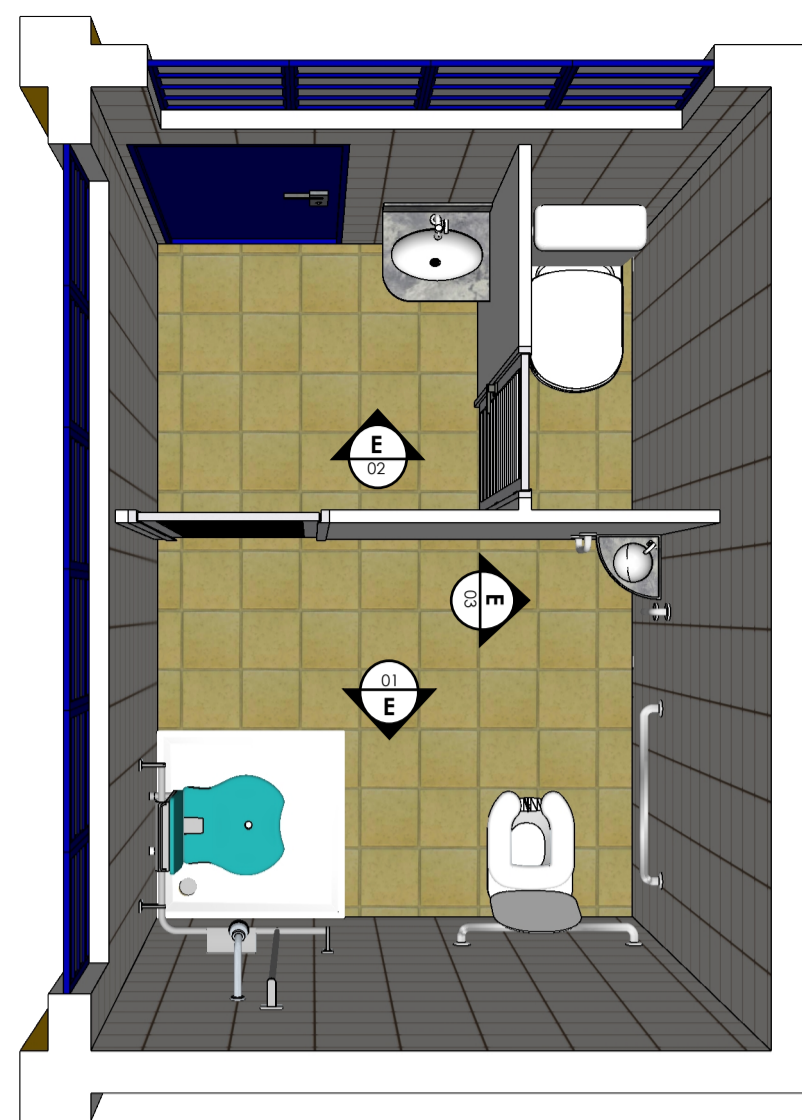
01 PLANTA BAIXA BANHEIRO FEMININO ESCALA 1/50
