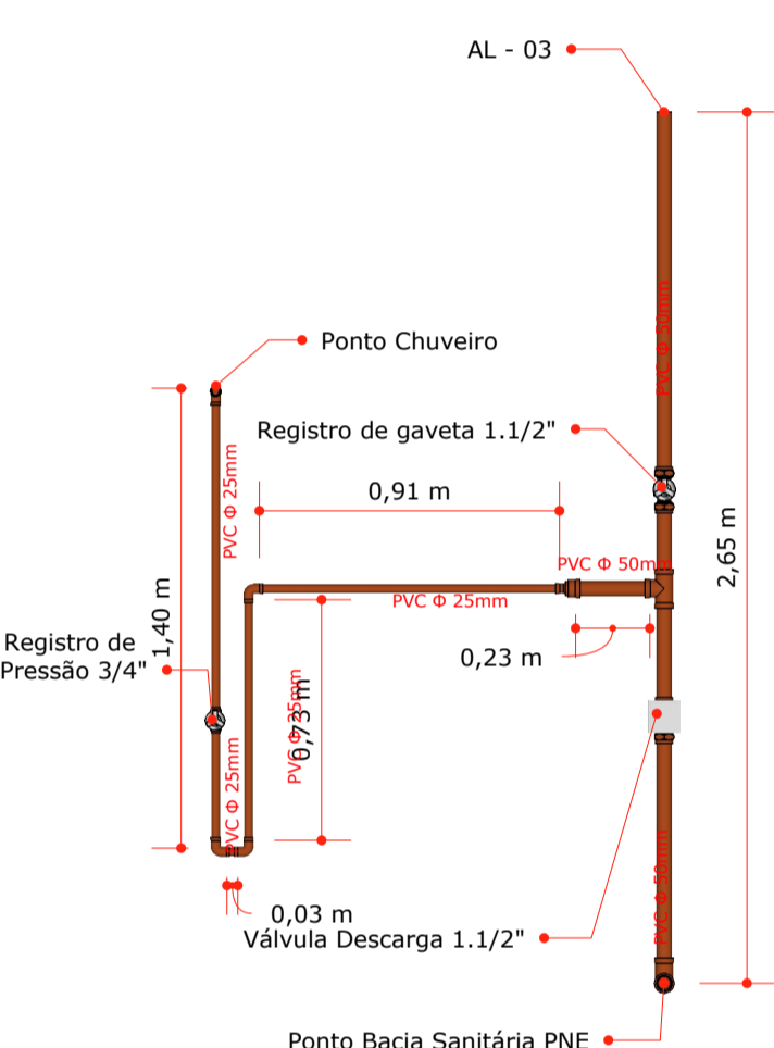
09 ELEVAÇÃO 04 - ÁGUA FRIA ESCALA 1/50
